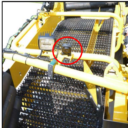
Caméra numérique peignes circulaires 1 et 2
