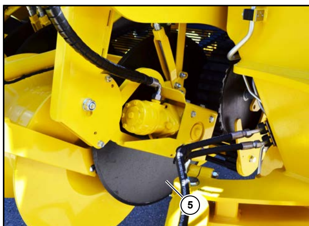
(5) Table de ramassage de butte avec coutres circulaires à entraînement hydraulique à gauche
