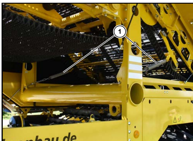
(1) Tendeur de chaîne de tamisage
