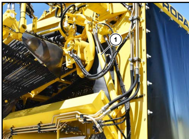
(1) Vérin inclinaison tapis à tétines 1/2
