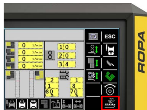
Touche programmable Table de visite avec option Roue motrice
