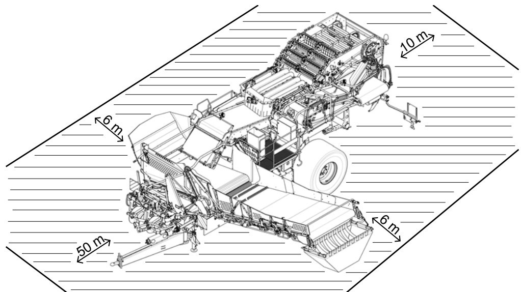
Zone de danger de la machine à trémie avec bras de chargement
