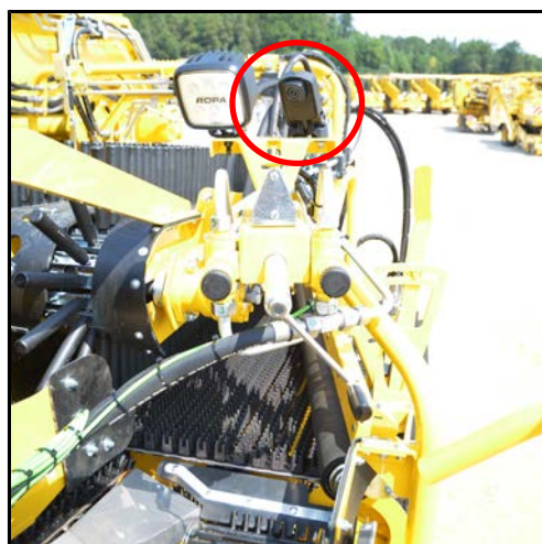
Caméra numérique tapis à déchets DoubleSelect
