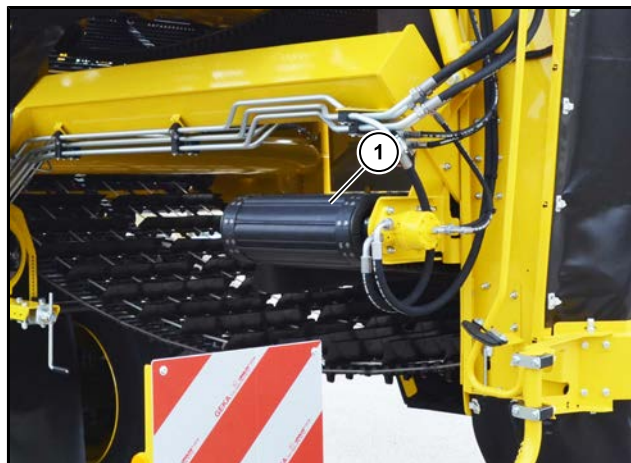
(1) Tapis d'évacuation de la saleté
