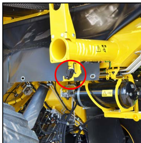
Caméra numérique tapis d'évacuation de la saleté
