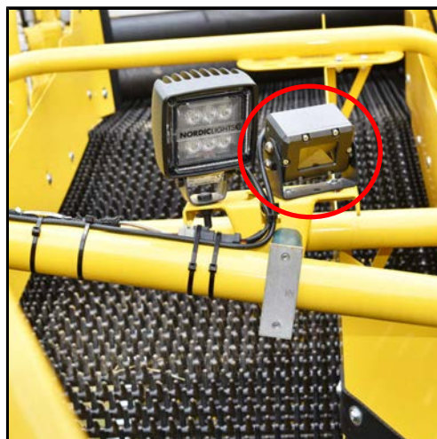
Caméra vidéo tapis à tétines 1/2
