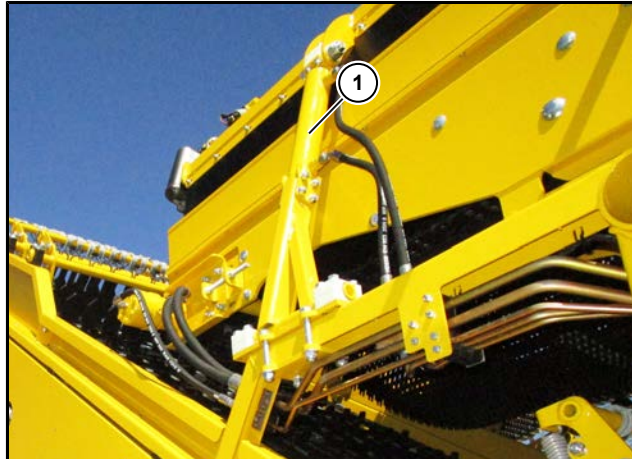
(1) Vérin inclinaison tapis à têtes 4
