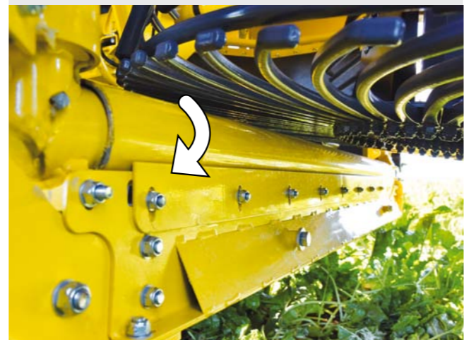
环形升降带入口处的旋转过渡管可防止积土
