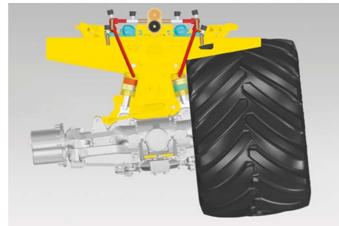
液压行走机构，自动斜坡平衡
