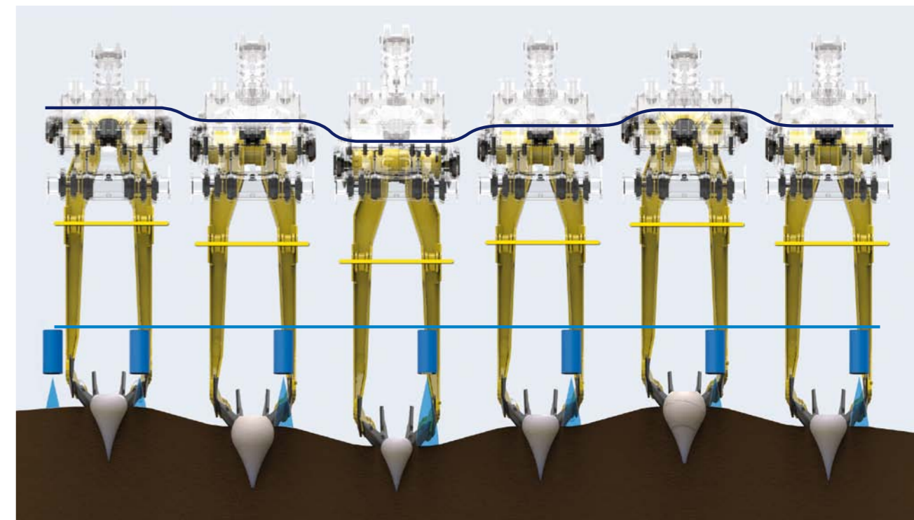
地面轮廓不平整时的犁刀深度自动调节 每个甜菜行旁的超声波传感器探测土地表面轮廓
