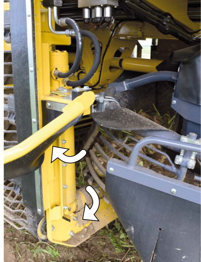
环形升降带入口处的旋转过渡管可防止积土
