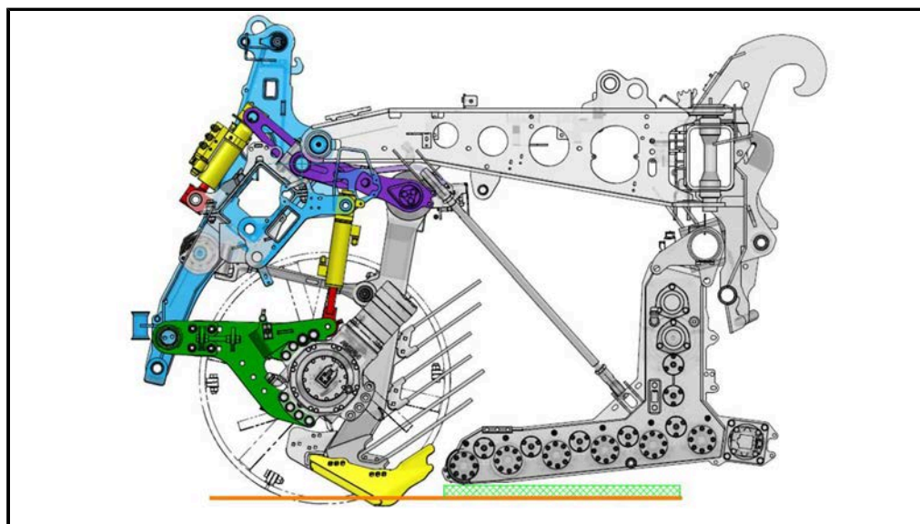
辊筒组处于较低位置
