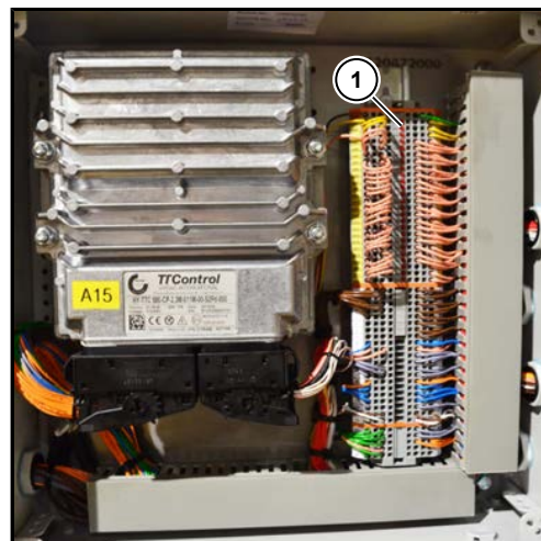
LED 在割台电气箱内
