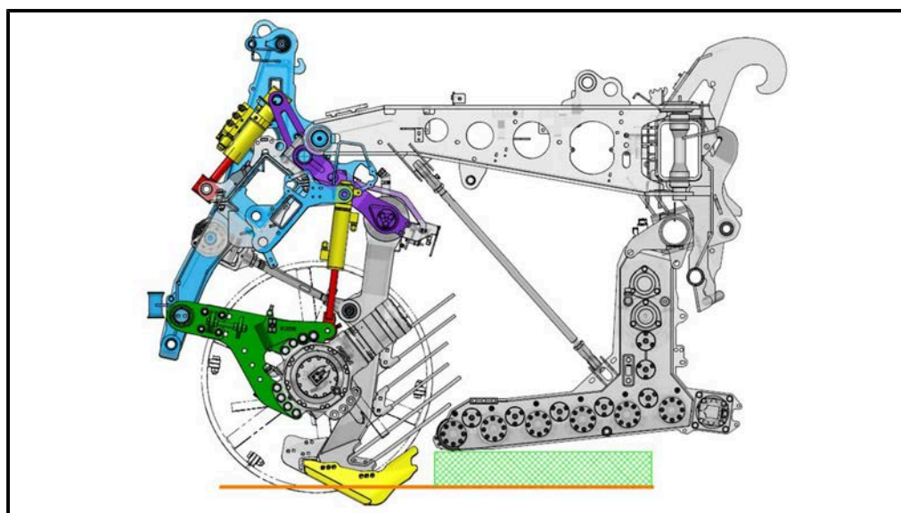
辊筒组处于较高位置
