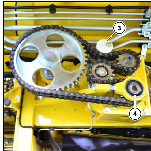
纵向刮板的驱动链
