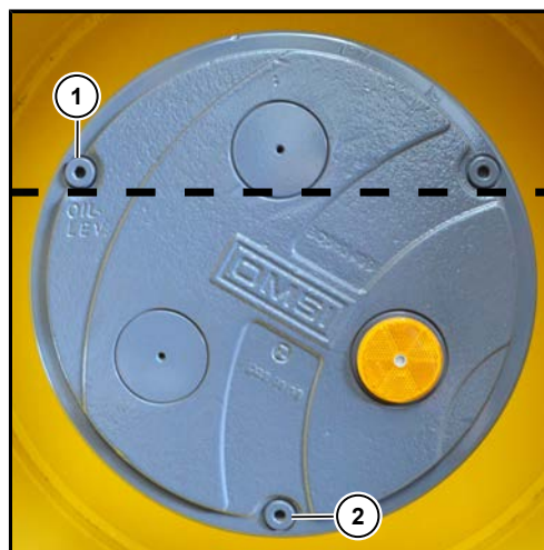
中后轴的行星传动机构
