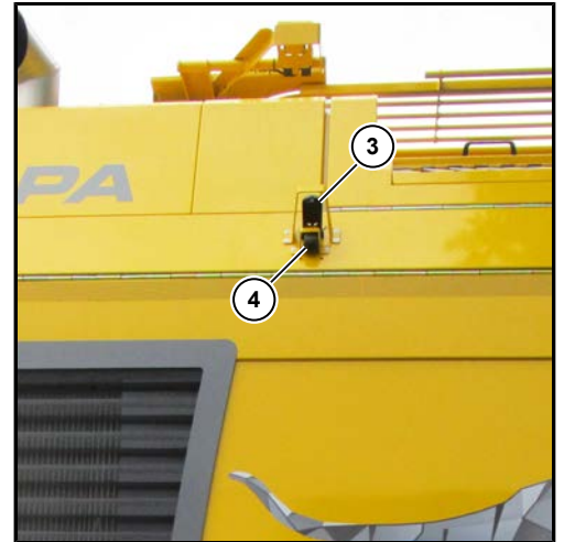
(3) 倒车摄像头 (4) 后方 R-View 摄像头
