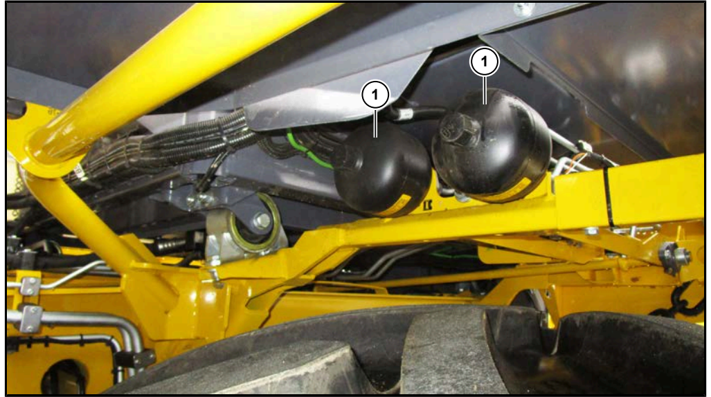
制动装置蓄压器
