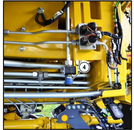
(4) 星状过滤网摄像头旁的压缩空气连接处
