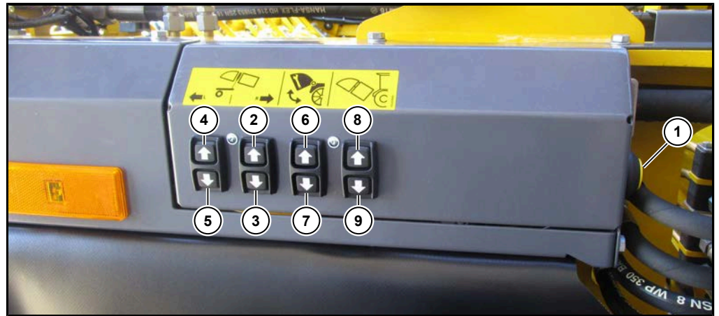
左侧犁头单元地面操作装置
