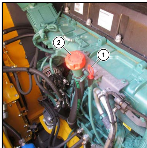
(1) 油标尺 (2) 加油盖
