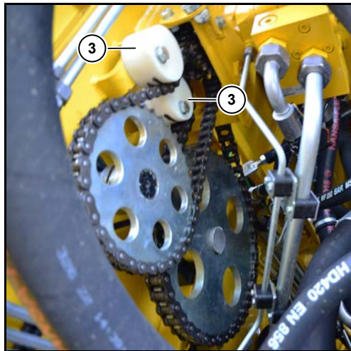
横向刮板和清洁辊筒的驱动链
