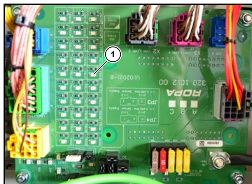
LED 在总电气装置
