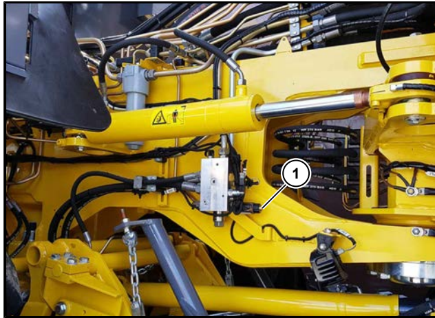
(1) Styrblock siktband
