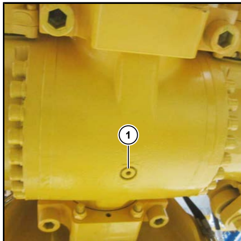
(1) Oljeavtappningsskruv
