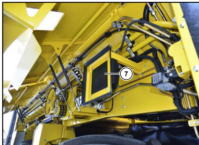
(7) Oljekylare tillsatsväxellåda
