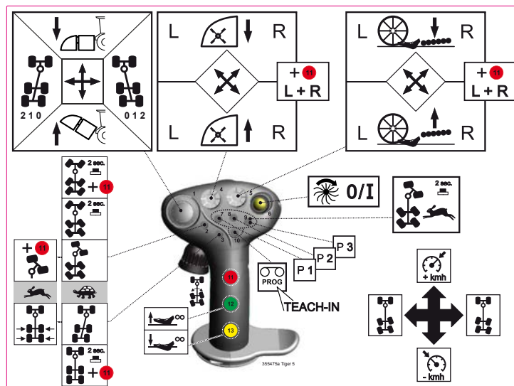
Joystickens baksidan
