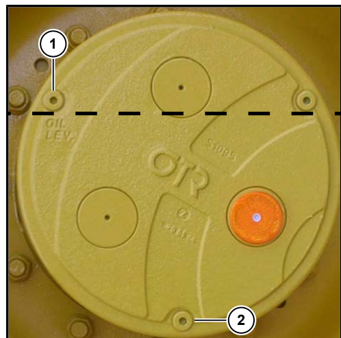
Rotismo epicicloidale asse posteriore
