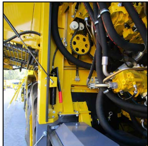
Supporto per ingrassatore a siringa
