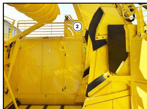
(2) Sensore a ultrasuoni posteriore
