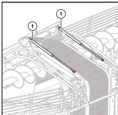
(1) Cilindri di supporto
