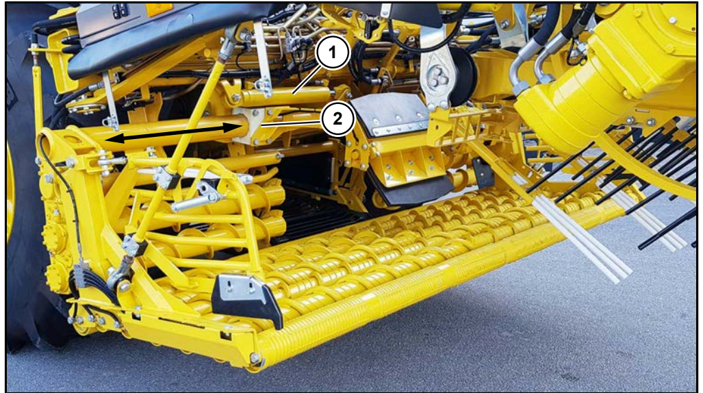
Passo rulli spostato verso destra Unità estirpatrice versione 2017
