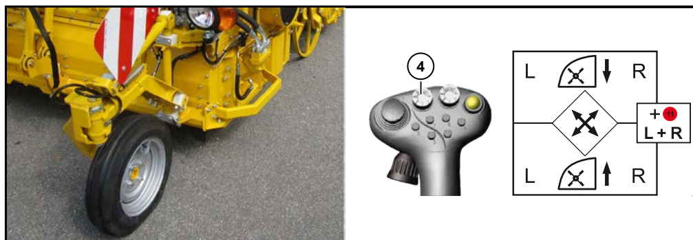
Ruota tastatrice in posizione di estirpatura
