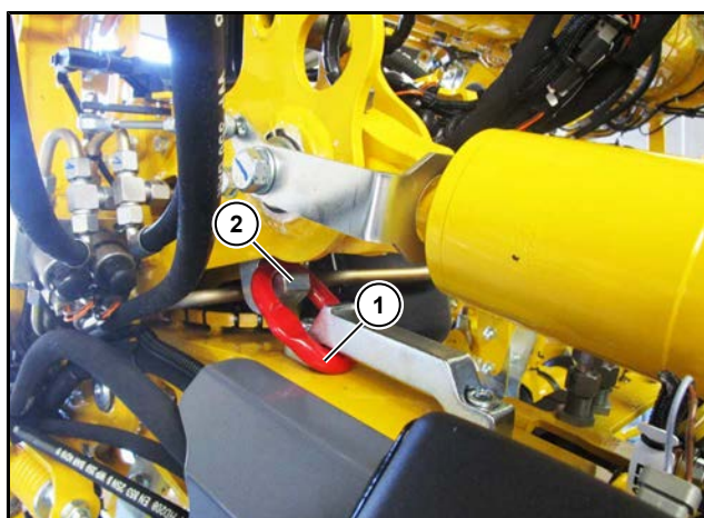
左侧止动件已挂上
