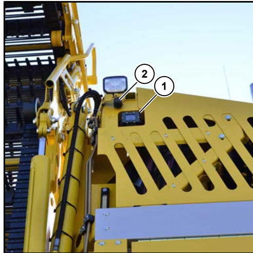
(1) 卸料带摄像头 (2) 左侧 R-View 摄像头
