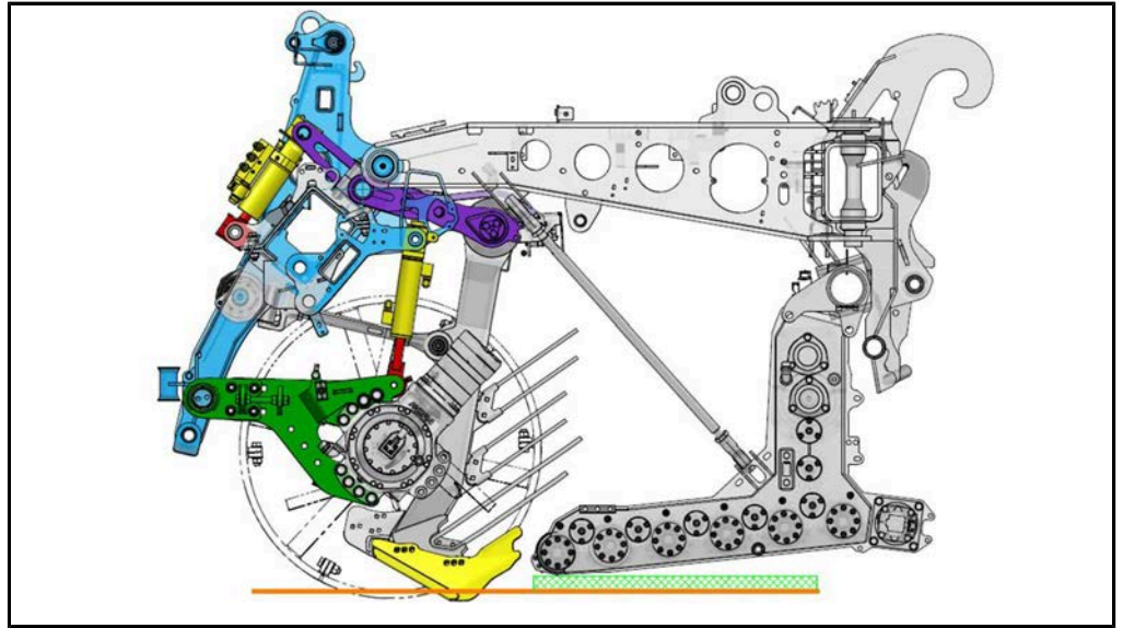
辊筒组处于较低位置
