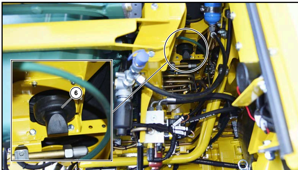
(6) 灰尘排出阀
