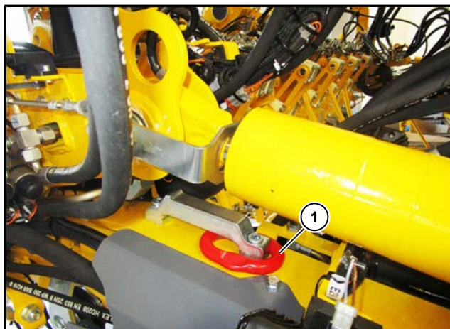
保存位置上的左侧止动件
