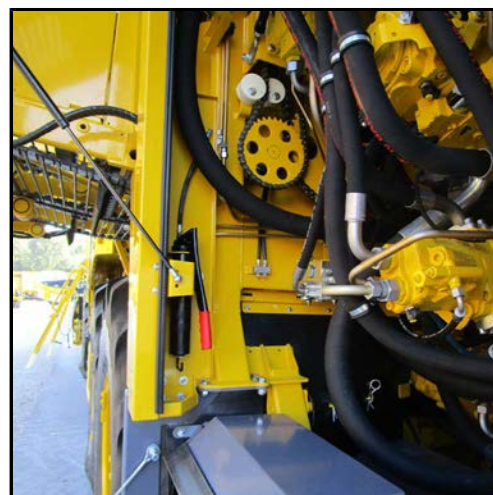
油枪的支架
