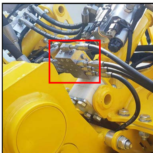
振动犁刀偏心轮驱动总分配器
