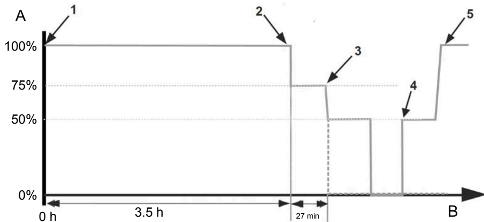
A 发动机扭矩 B 时间轴
