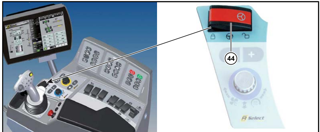
(44) 转向控制总开关
