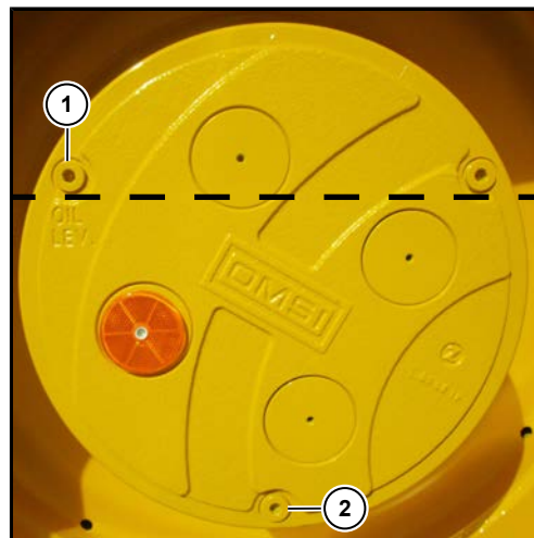
行星传动机构前轴
