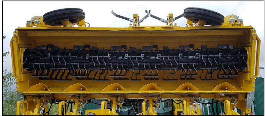
RIS 型打叶器轴
