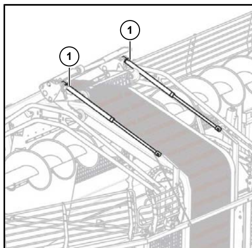
(1) 支撑油缸
