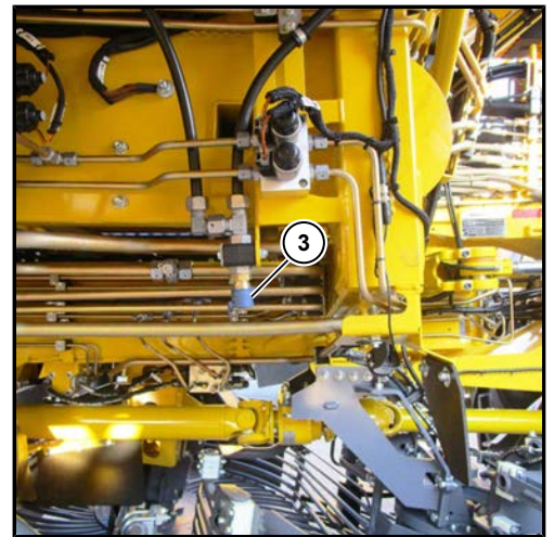
(3) 星状过滤网摄像头旁的压缩空气连接处
