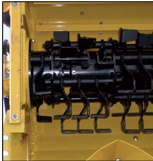
RIS 上的打叶器刀和夹紧搭板
