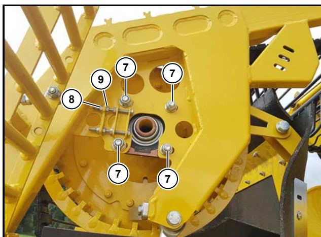
Imaginea ilustrează reglarea elevatorului la partea dreaptă, față
