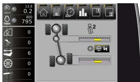
Indicador treaptă de viteză pentru virare la dreapta activă
