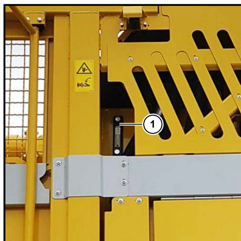
(1) Vizor de control nivel de ulei + temperatură ulei
