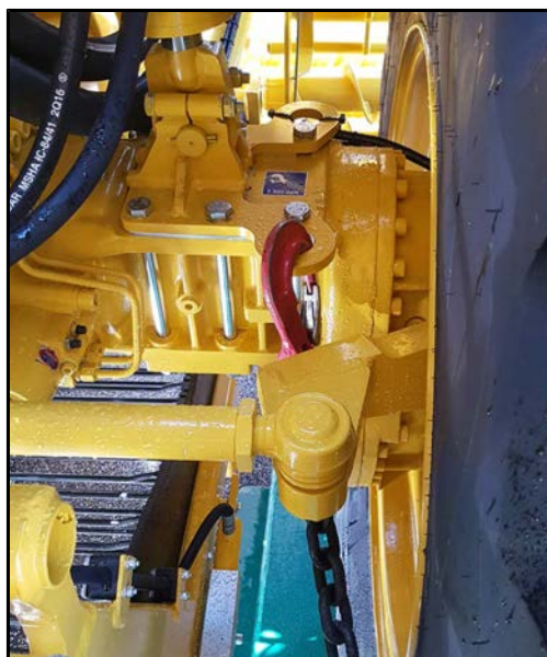
Urechi de ancorare la osia față
