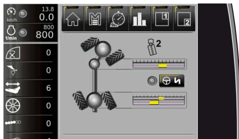
Indicador în cazul funcției de întoarcere activă vezi Pagina 212
