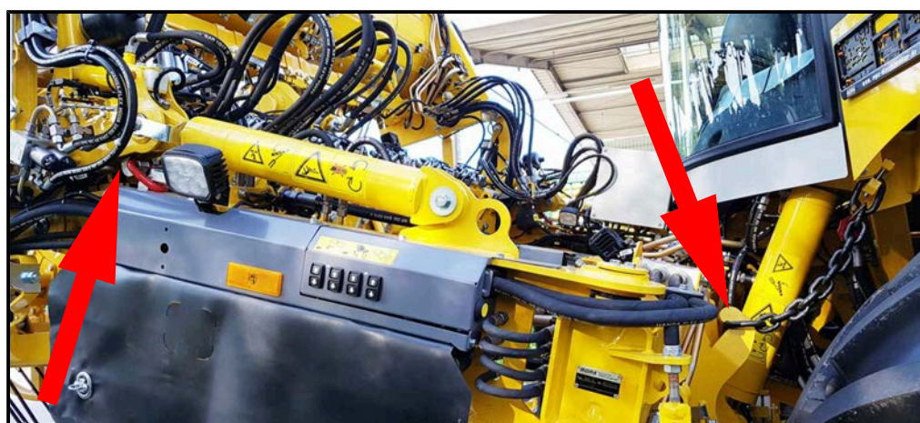
Mașină de tăiat frunze în poziție de întreținere
