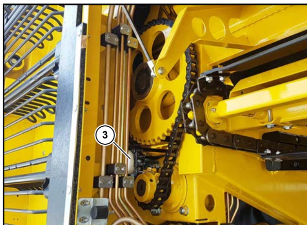
Lanț de acționare transportor cu racleți longitudinali
