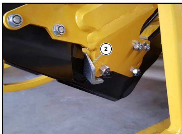
Cornierul de uzură (2) folosește la protejarea suportului brăzdarului împotriva frecării. Înlocuiți cornierul de uzură, înainte să își piardă funcția de protecție!
