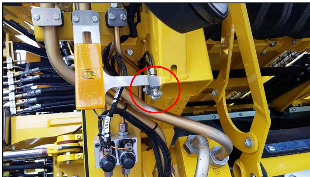
Bloc niplu de lubrifiere la angrenajul transportorului cu racleți transversali
