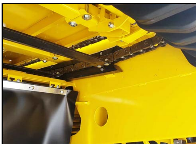
Corecți tensionarea lanțului
