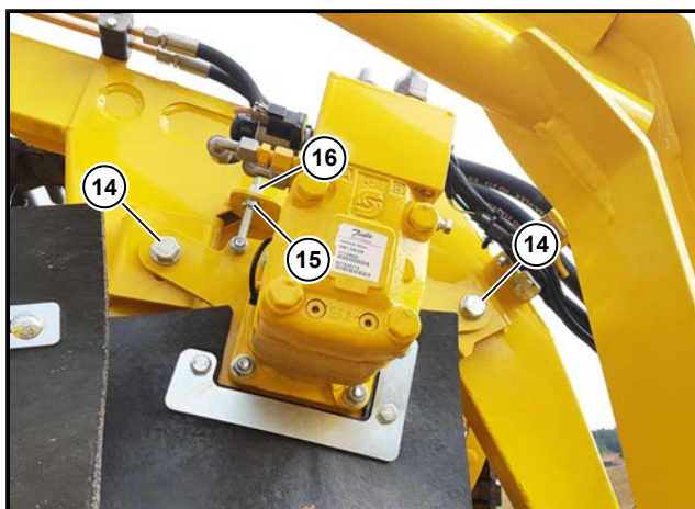
Imaginea ilustrează elevatorul dreapta spate
