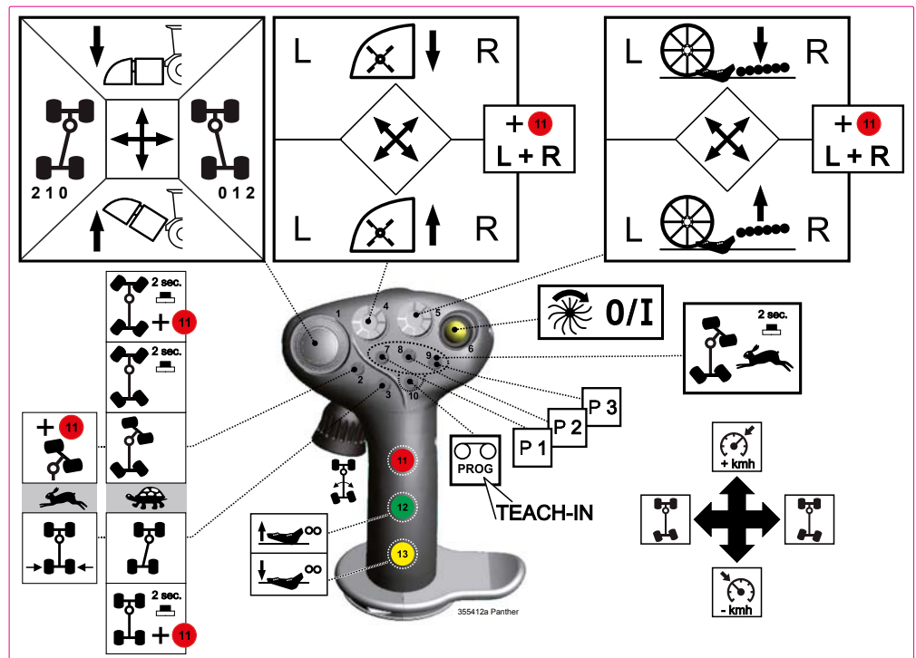
Partea din spate a joystick-ului
