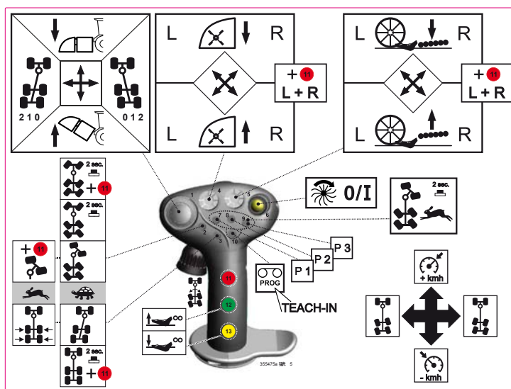
操纵杆背面
