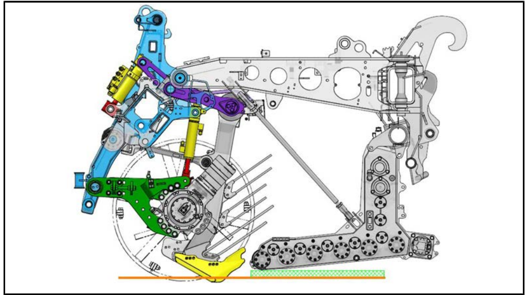
轱筒组处于较低位置
