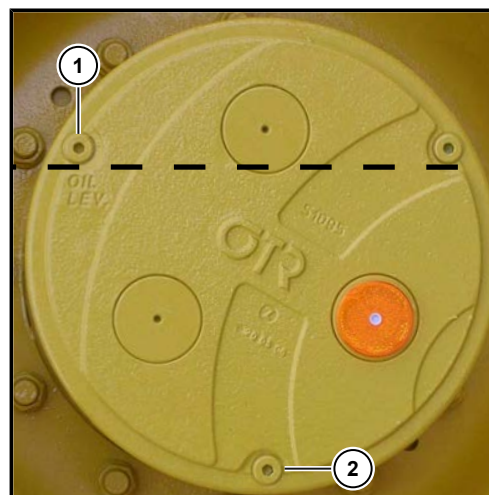
行星传动机构后轴
