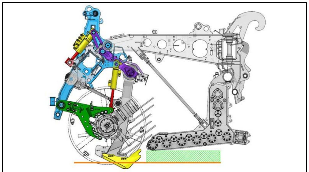
轱筒组处于较高位置
