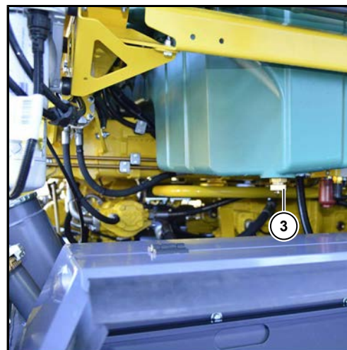
(3) 发动机排油阀
