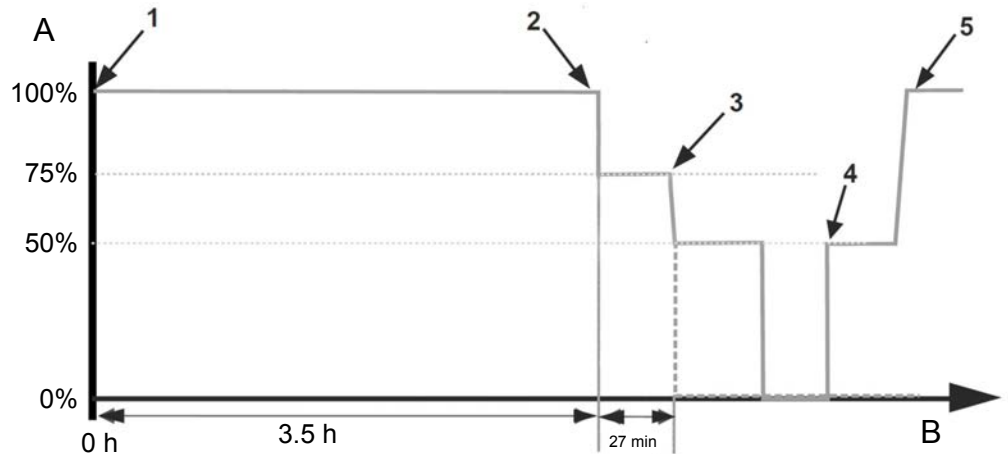
A 发动机扭矩 B 时间轴
